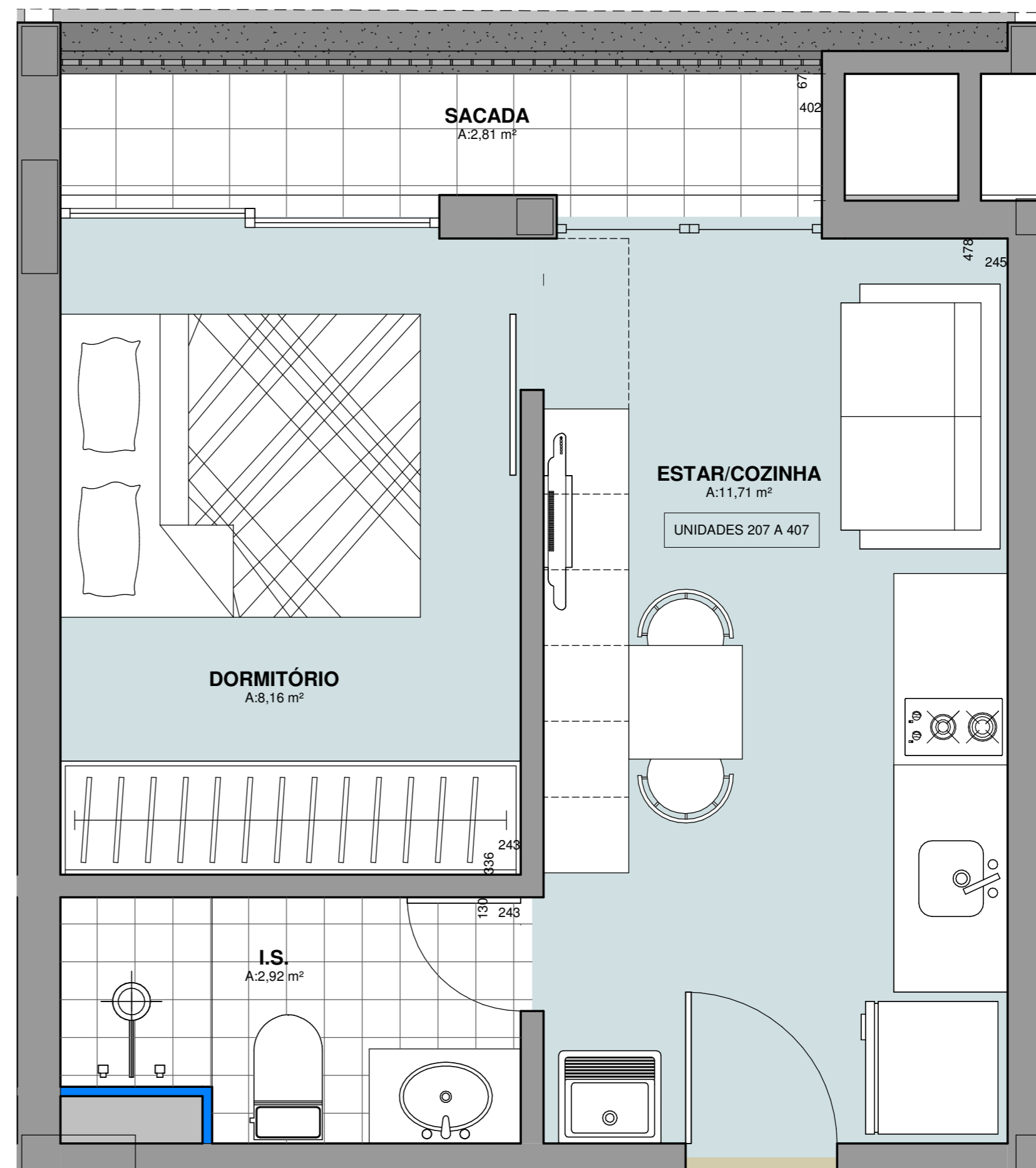
UNIDADE TIPO - 207 A 407
